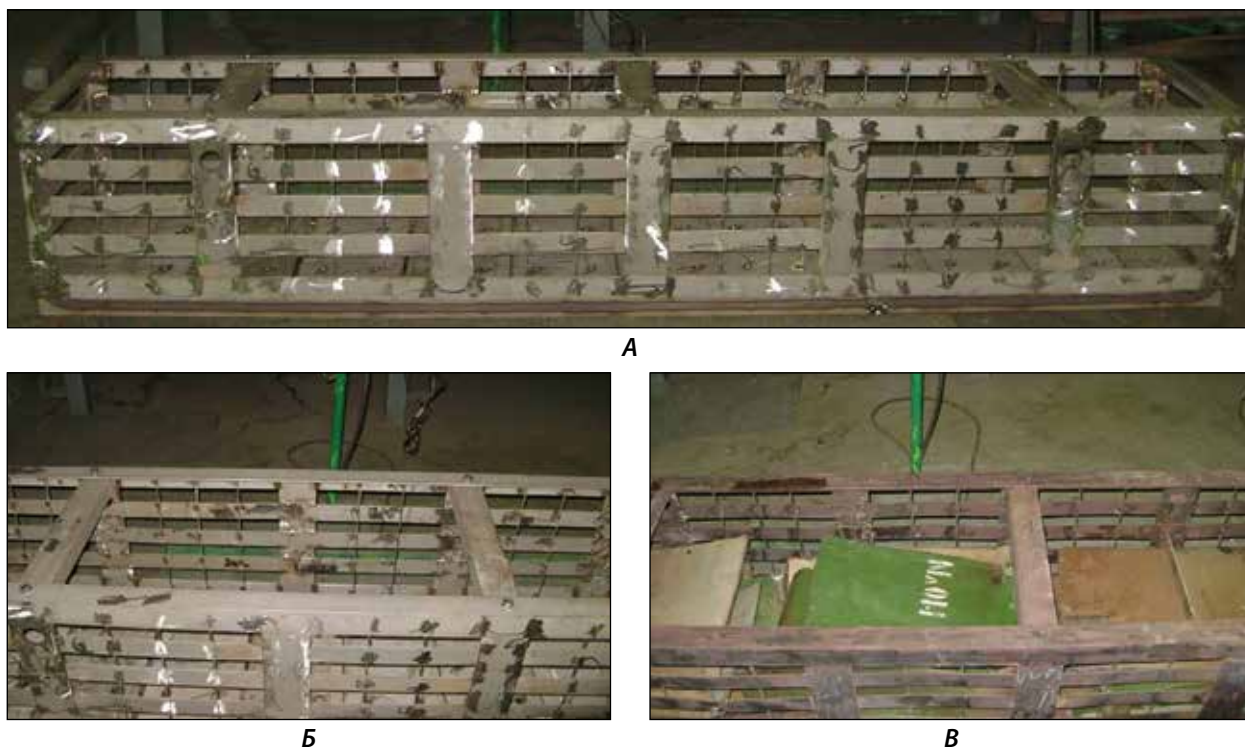
Рисунок 3 – Поддоны, использовавшиеся в процессе прокаливания фрагментов металлоконструкций: А – общий вид поддона; Б – взвешивание пустого поддона; В – взвешивание поддона с фрагментами металлоконструкций (март 2017 г., фотографии авторов)
