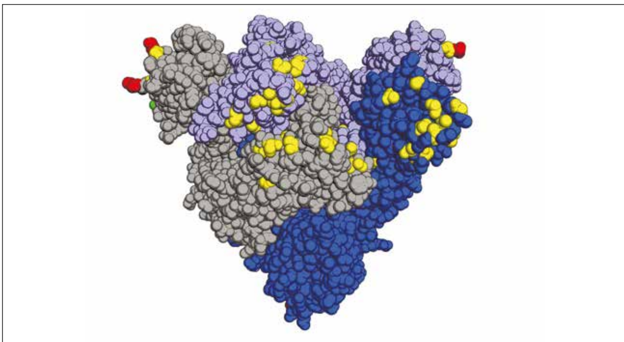
Рисунок 1 – Схема расположения мутаций белка S варианта омикрон вируса SARS-CoV-2. Представлен пример S-белка варианта омикрон вируса SARS-CoV-2 (вид сверху). В тримерной структуре два мономера выделенные серым и светло-фиолетовым цветом содержат свои рецептор-связывающие домены (Receptor-Binding Domain, RBD) в «нижней» конформации, мономер, выделенный темно-синим цветом, содержит RBD в «верхней» конформации. 2. Аминокислотные замены по сравнению с исходным штаммом выделены желтым, делеции – красным, вставки – зеленым цветом [10]
